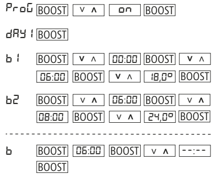
Obr. 3: Příklad programování
