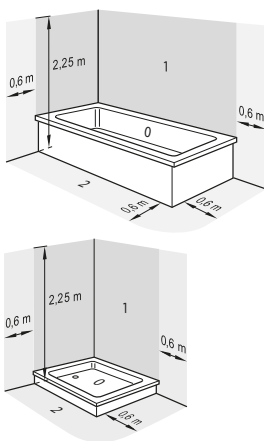
Abb. 1: Schutzbereichseinteilung
