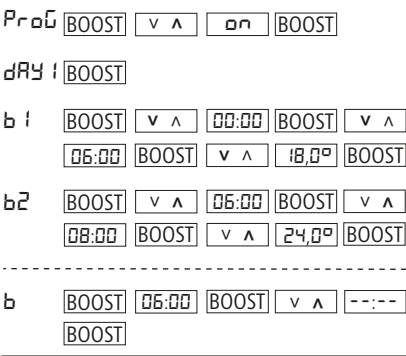
Rys. 3: Przykładowe programowanie
