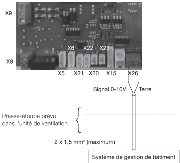
Circuit imprimé D275 III
