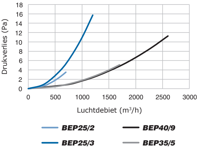
Drukverlies BEP
