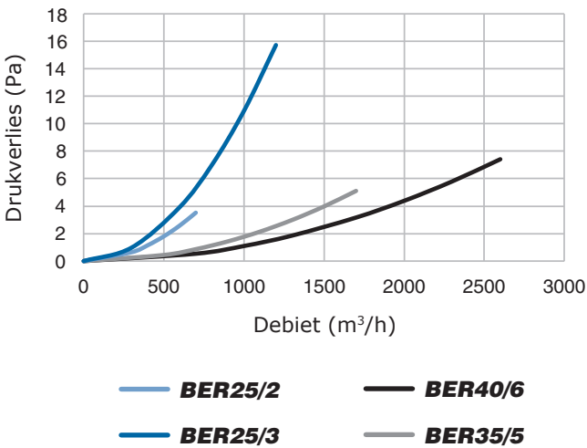
Drukverlies BER
