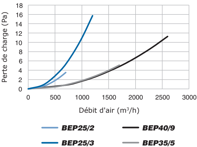
Perte de charge BEP
