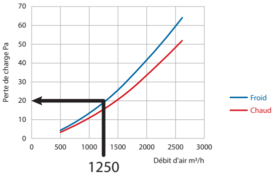
Perte de charge côté air ENY-P3/P4
