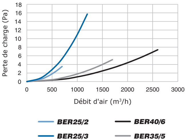
Perte de charge BER
