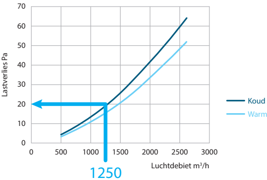
Luchtzijdig drukverlies ENY-P3/P4
