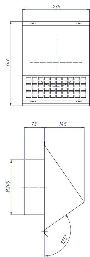
Grille de sortie murale Ø 255/200
