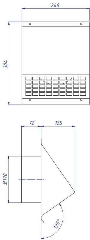
Grille de sortie murale Ø 200/170
