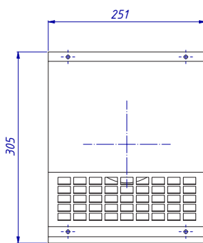
Grille de sortie murale 160/125 mm
