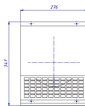
Grille de sortie murale 255/200 mm
