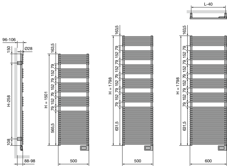
HR-EL-A Hartafstand tussen de ophangingen L-40 H-258
