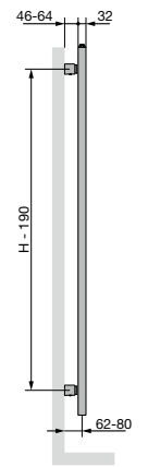
VUE LATÉRALE
