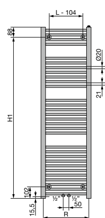
VUE ARRIÈRE
