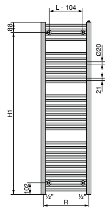
VUE ARRIÈRE
