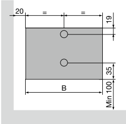
Universele aansluiting UN (standaard) | Zijaanzicht
