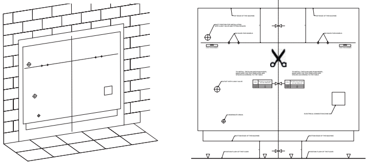
Installatiesjabloon
