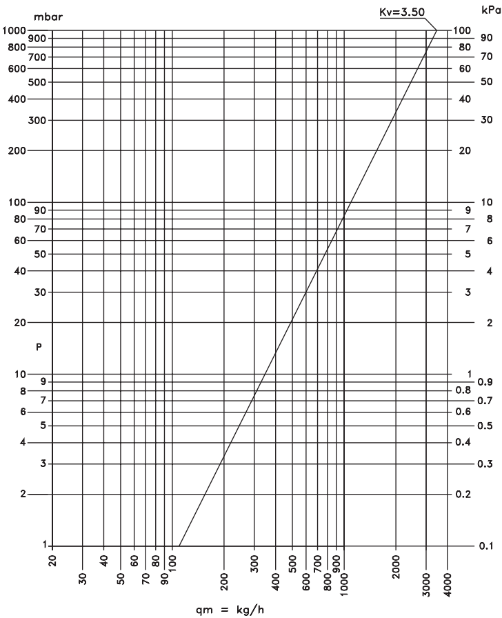
Diagramm mit Lastverlusten bei vollständig geschlossenem 3-Wege-Ventil.
