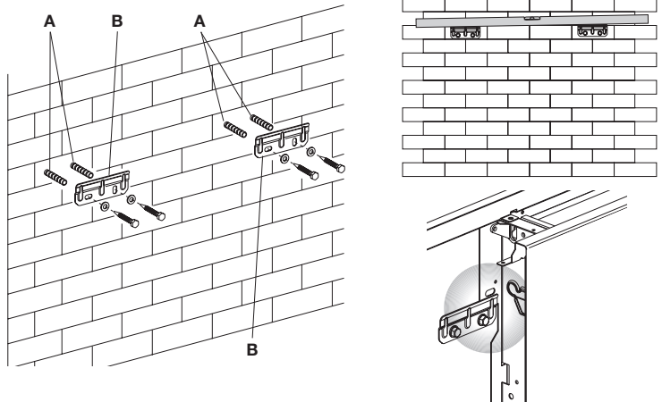
Beugels
