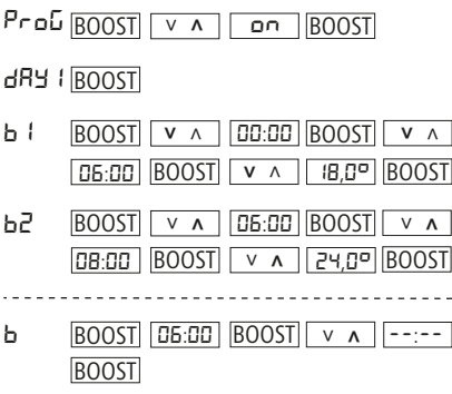
Obr. 3: Příklad programování
