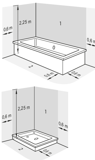
Fig. 1: Indeling veiligheidszones
