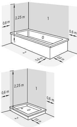
Abb. 1: Schutzbereichseinteilung
