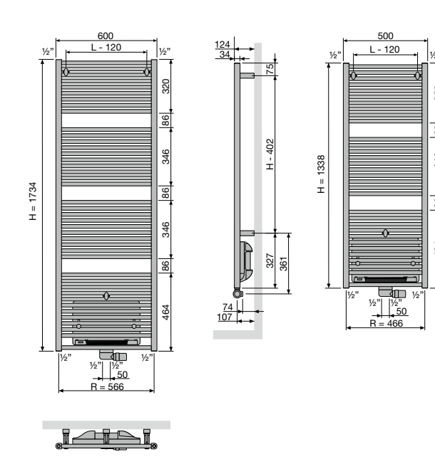
HDM-BL-MIX Hartafstand tussen de ophangingen L-120 H-402
