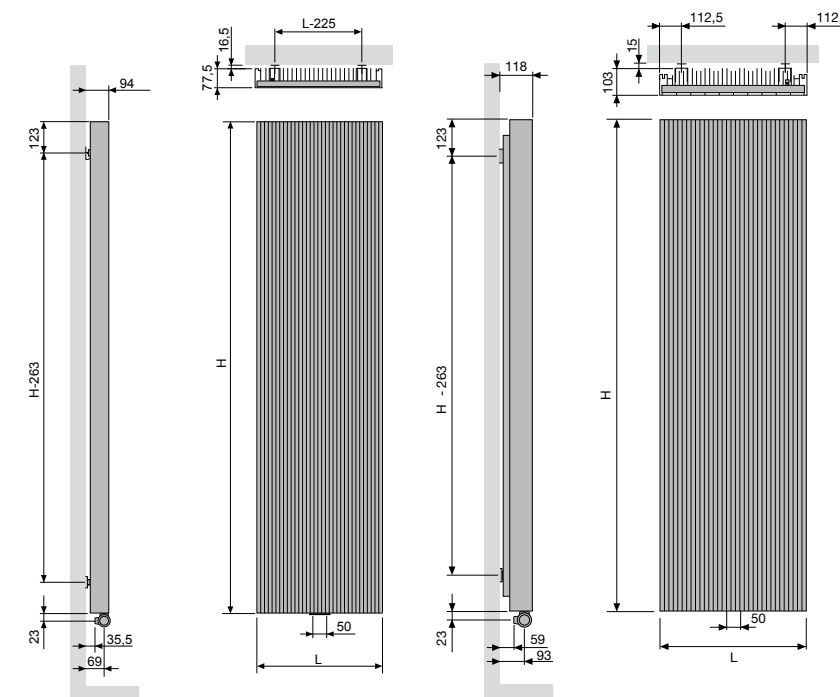
BRYCE V75 / BRYCE V100 Hartafstand tussen de aansluitingen 50 Hartafstand tussen de ophangingen L-225
