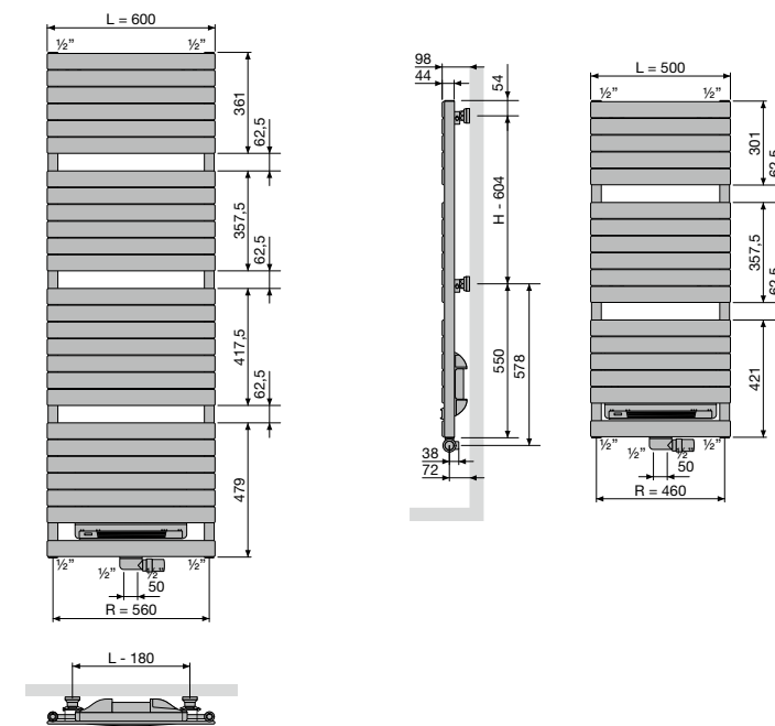
HF-BL-MIX Hartafstand tussen de ophangingen L-180 H-604
