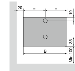
Universele aansluiting UN (standaard) | Zijaanzicht
