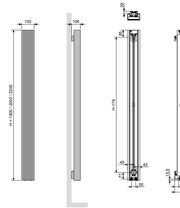
BRYCE MONO Hartafstand tussen de aansluitingen 50
