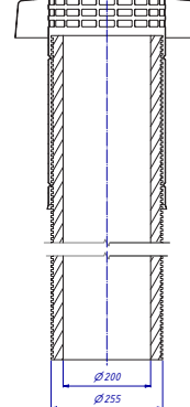
A-A ( 1/5 )
