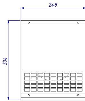
Geveldoorvoer 200/170 mm
