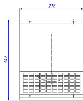
Geveldoorvoer 255/200 mm
