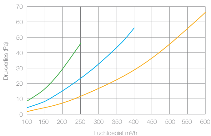
Toevoer (aanzuig)
