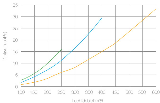
Afvoer (uitblaas)
