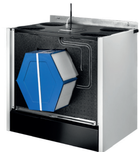
Toegang tot warmtewisselaar, ventilatoren en elektronica
