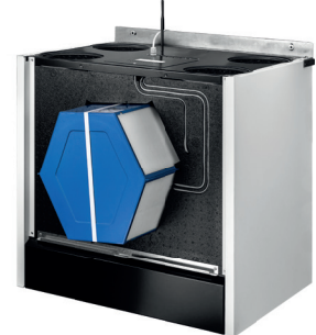
Accès à l'échangeur de chaleur, aux ventilateurs et à l'électronique
