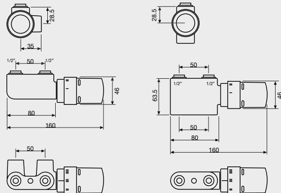
ECKAUSFÜHRUNG DESIGN-VENTILGARNITUR
