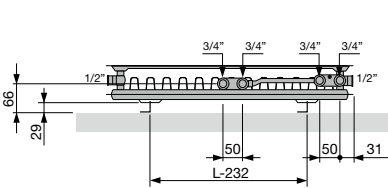
ONDERAANZICHT T21S
