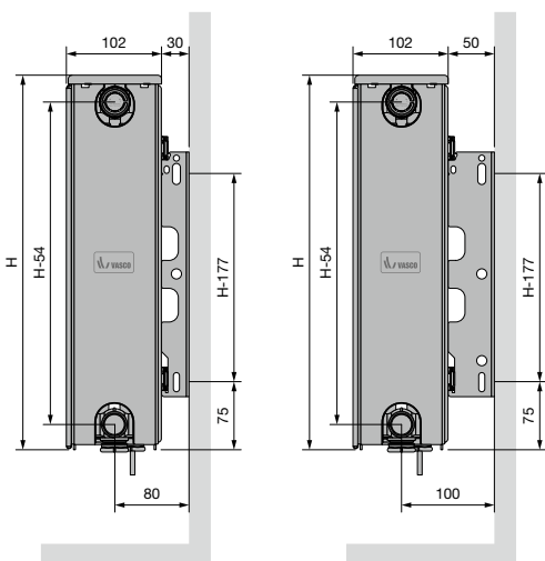
ELIA 8D (TYPE 22) VLAKKE VOORZIJDDE, ELIA 8L (TYPE 22) GELIJNDE VOORZIJDDE
