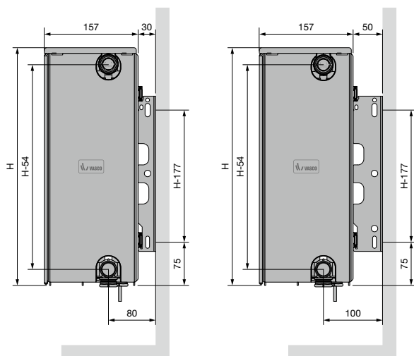
ELIA 8D (TYPE 33) VLAKKE VOORZIJDDE, ELIA 8L (TYPE 33) GELIJNDE VOORZIJDDE
