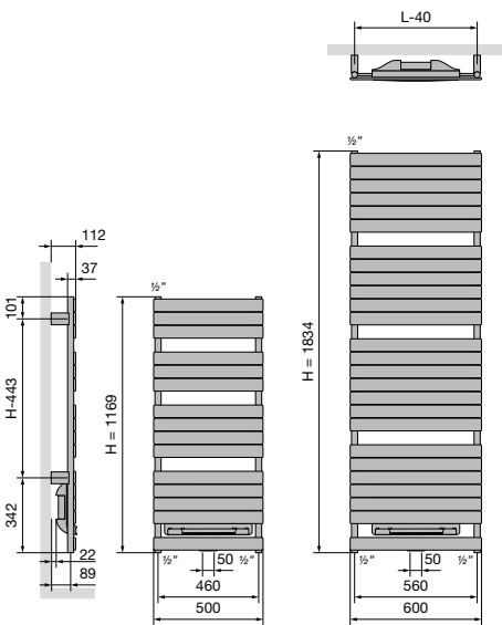
HF-BL-MIX-A Hartafstand tussen de ophangingen L-40 H-443
