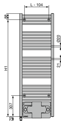
ACHTERAANZICHT
