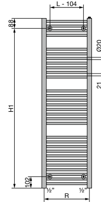
ACHTERAAZICHT
