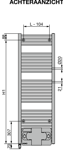
ACHTERAANZICHT
