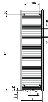
ACHTERAAZICHT
