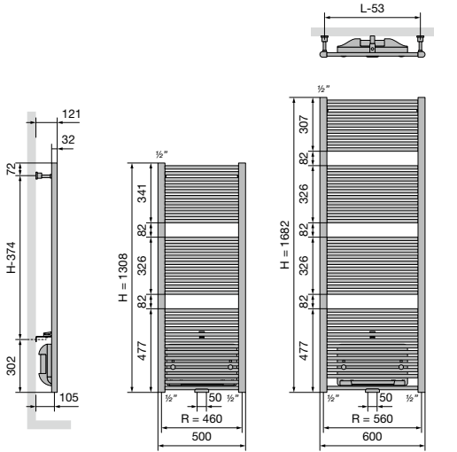
HDM-BL-MIX-A Hartafstand tussen de ophangingen L-53 H-374
