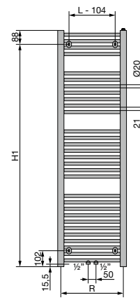
ACHTERAANZICHT
