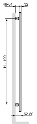
ZIJAAANZICHT
