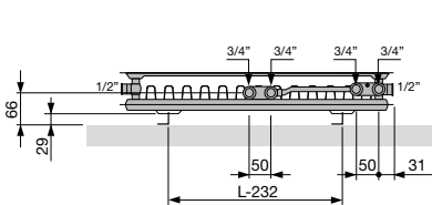
ONDERAANZICHT T21S
