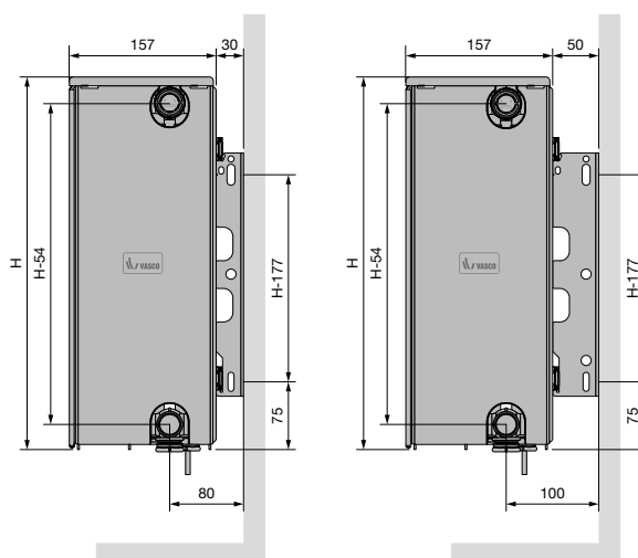
ELIA 8D (TYPE 33) VLAKE VOORZIJDE, ELIA 8L (TYPE 33) GELIJNDE VOORZIJDE
