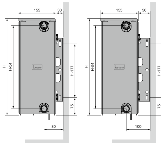
ELIA 4K (TYPE 33) PROFIEL VOORZIJDE
