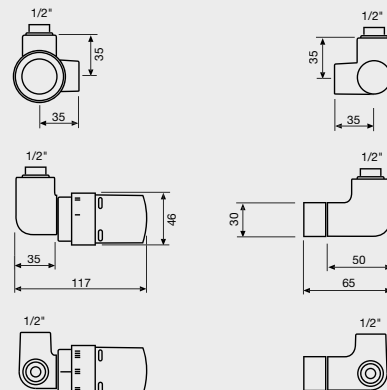
VENTIELSET 1-8
