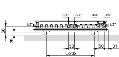
ONDERAANZICHT T21S
