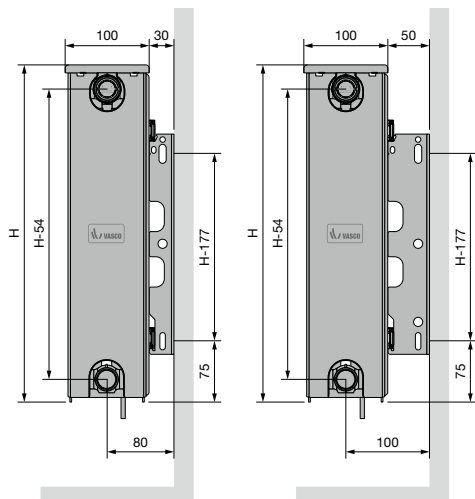
ELIA 4K (TYPE 22) PROFIEL VOORZIJDE
