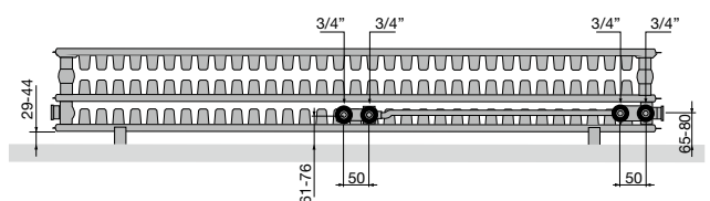
T33 | Onderaanzicht
