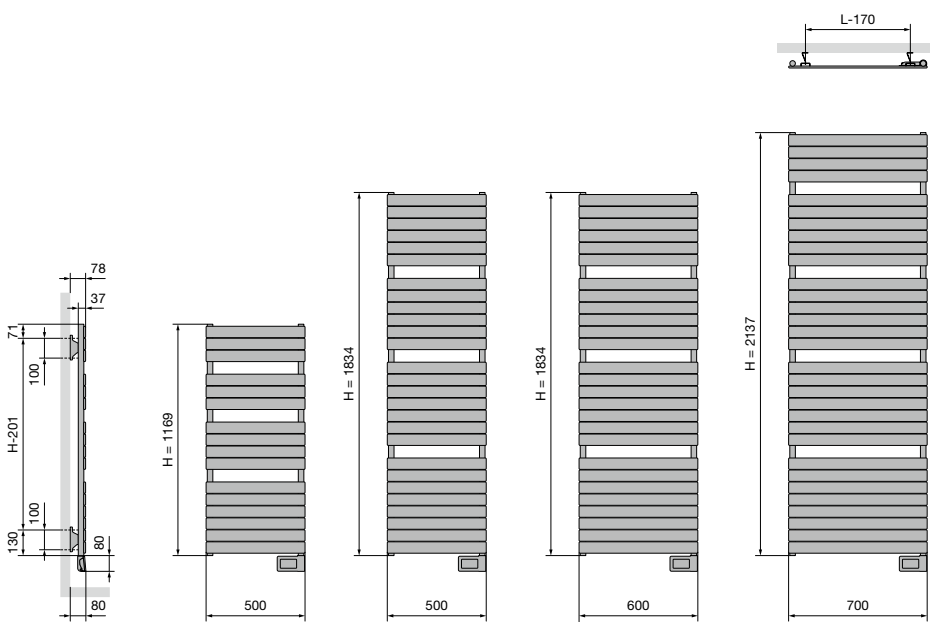
HF-EL-A Hartafstand tussen de ophangingen L-170 H-201
