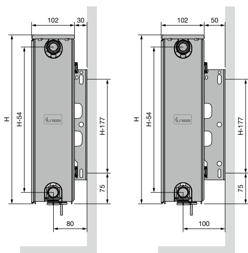
ELIA 8D (TYPE 22) VLAKE VOORZIJDE, ELIA 8L (TYPE 22) GELIJNDE VOORZIJDE
