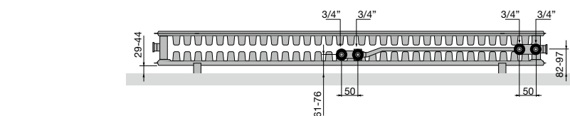
T22 | Onderaanzicht
