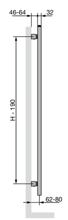
ZIJAAANZICHT
