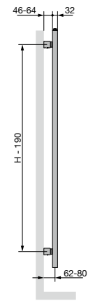
ZIJAAANZICHT
