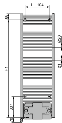
ACHTERAANZICHT
