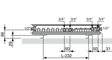
ONDERAANZICHT T21S
