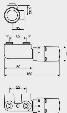
HAAS DESIGN-VENTIELSET
