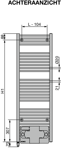
ACHTERAANZICHT
