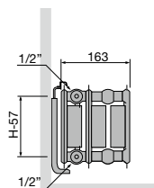
T33 | Zij aanzicht
