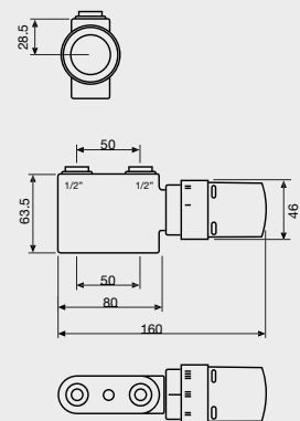
RECHT DESIGN-VENTIELSET
