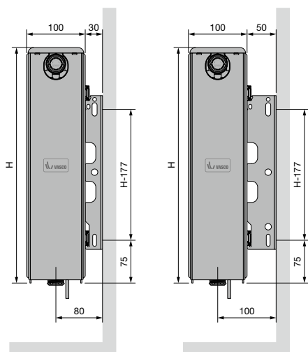
ELIA 5U (TYPE 22) PROFIEL VOORZIJDE
