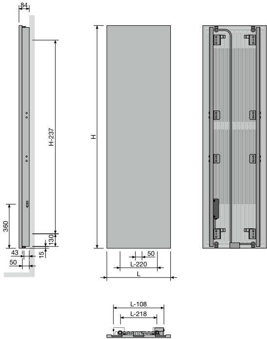
N1L1-EL-MIX
