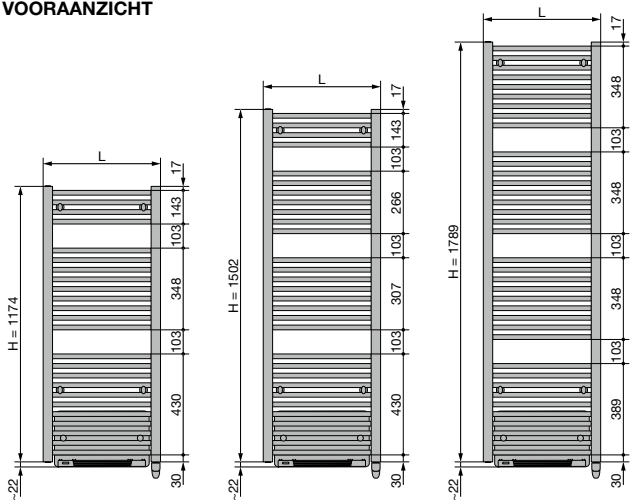
VOORAANZICHT
