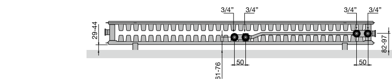
T22 | Onderaanzicht
