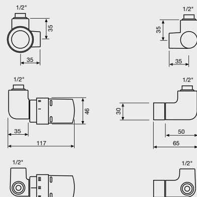
VENTIELSET 1-8
