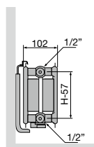
T22 | Zij aanzicht
