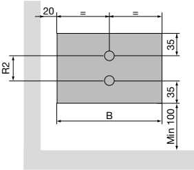
Aansluiting SL/SR | Zijaanzicht
