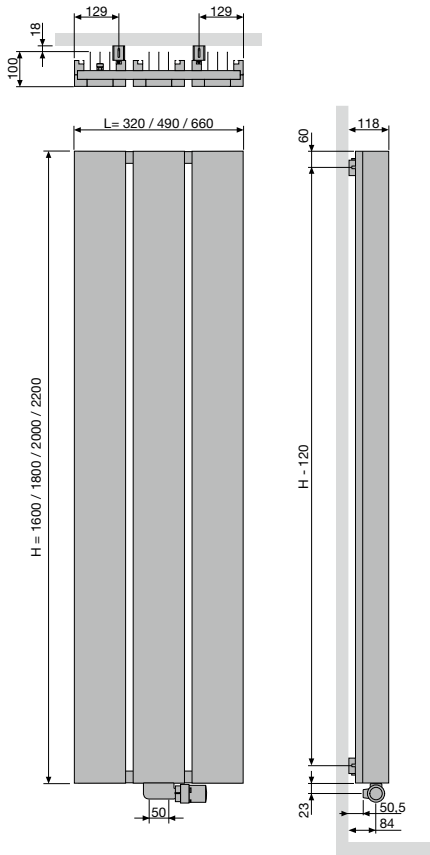
BEAMS Hartafstand tussen de aansluitingen 50 Hartafstand tussen de ophangingen L-258
