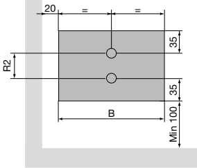
Aansluiting SL/SR | Zijaanzicht
