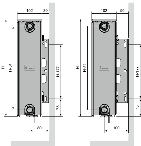
ELIA 8D (TYPE 22) VLAKE VOORZIJDDE, ELIA 8L (TYPE 22) GELIJNDE VOORZIJDDE
