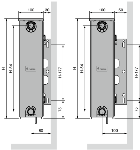
ELIA 4K (TYPE 22) PROFIEL VOORZIJDDE
