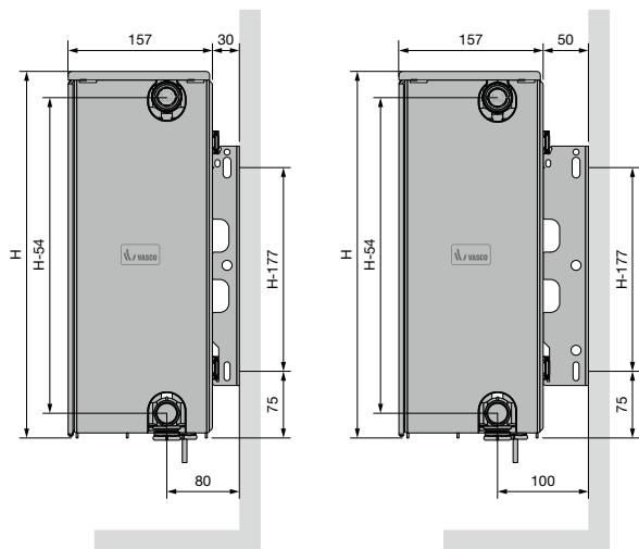
ELIA 8D (TYPE 33) VLAKE VOORZIJDDE, ELIA 8L (TYPE 33) GELIJNDE VOORZIJDDE
