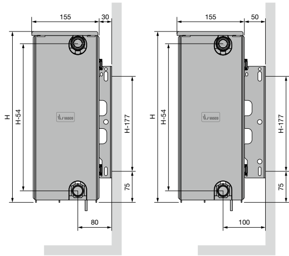
ELIA 4K (TYPE 33) PROFIEL VOORZIJDDE
