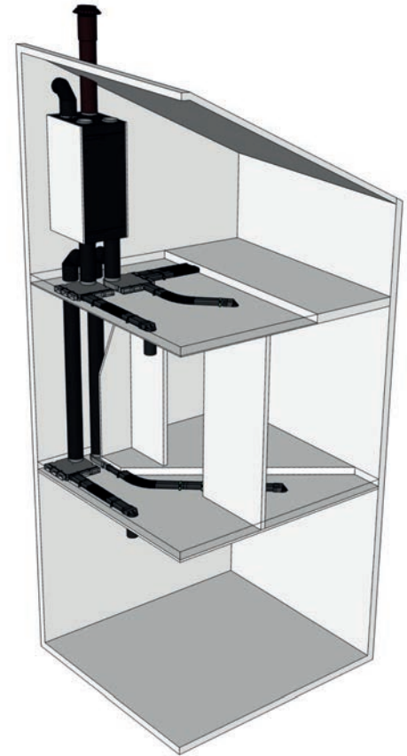
Balansventilatie (systeem D)
