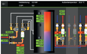
overzicht verwarmingssysteem
