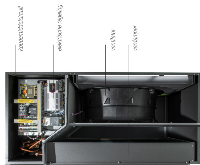
Opengewerkt bovenaanzicht
